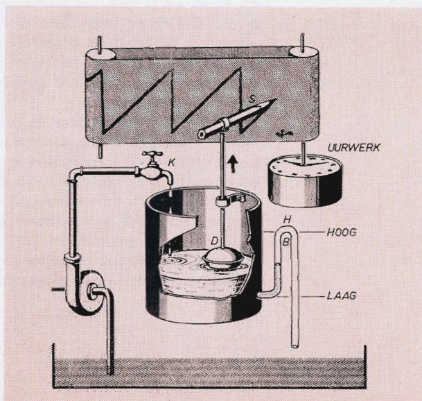
Fig. 15 Een hydraulische zaagtandgenerator
