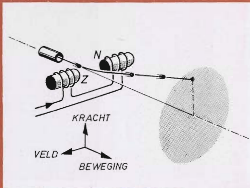
Fig. 9 Magnetische afbuiging
